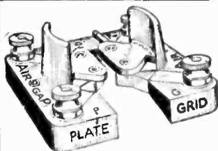
Type U. X. Universal Price 60c
